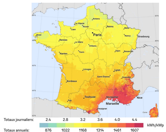
kWh produit par kW installé
